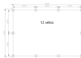
Abri Forêt 6m x 4m
