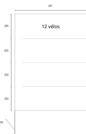
Abri 6m x 10m
