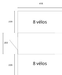
Abri 4m x 6m
