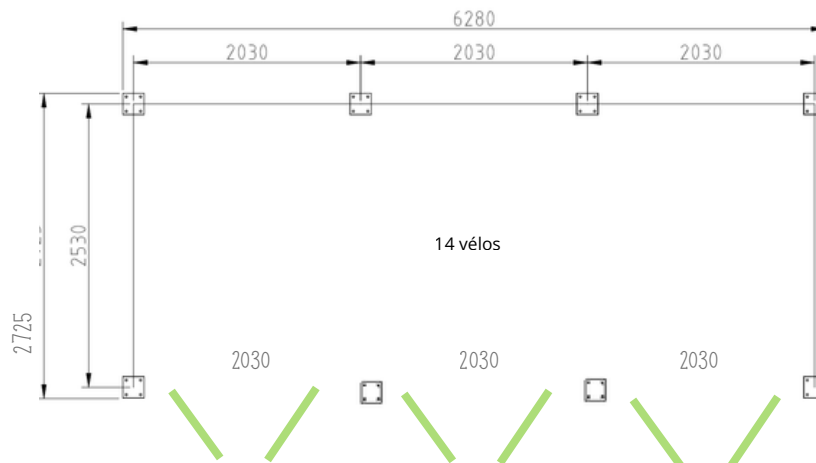
Abri lapiaz Compact 6m x 2,5m
